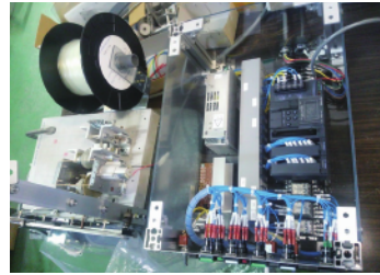
開発中のチューブ切断機
